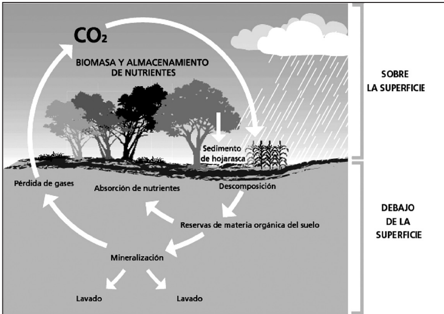
Figura 4. Procesos del ciclo de carbono en SAF
