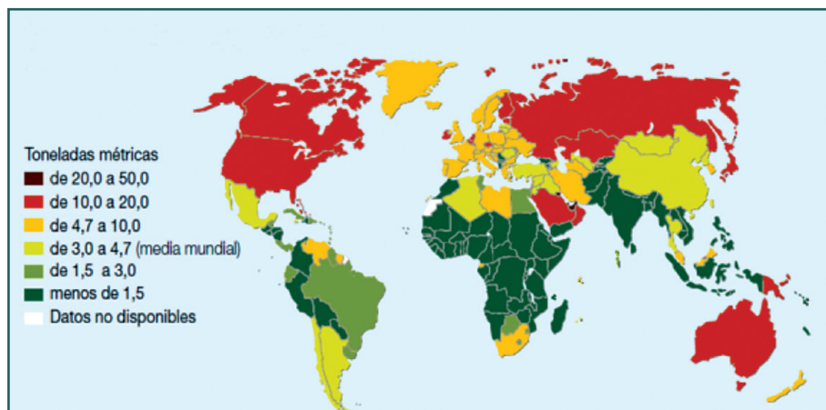
Figura 1. Emisiones de CO 2 per cápita (2006)
