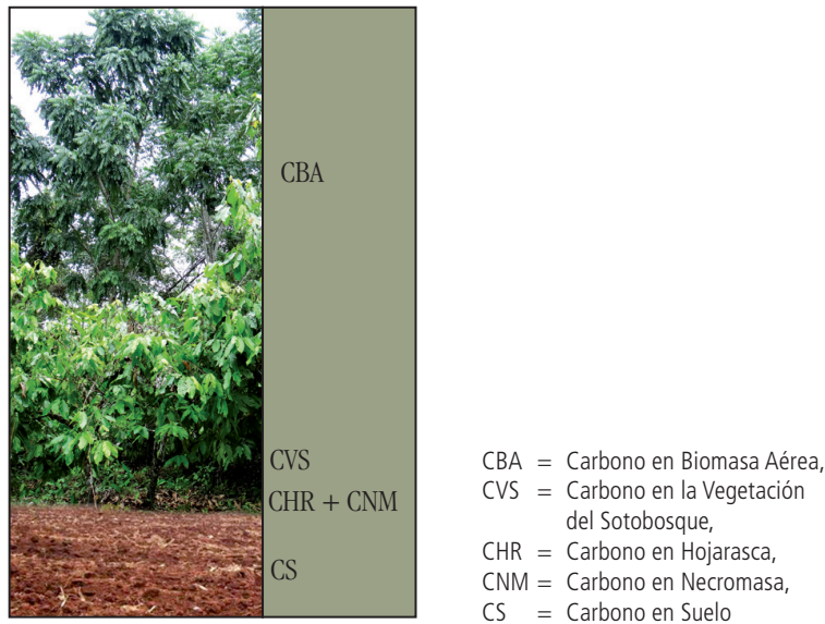
Figura 9. Depósitos de carbono en un sistema agroforestal
