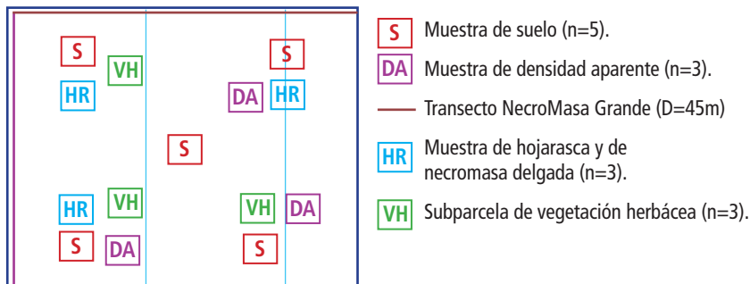
Figura 10. Muestra esquemática de la parcela de muestreo para la evaluación del SAF
